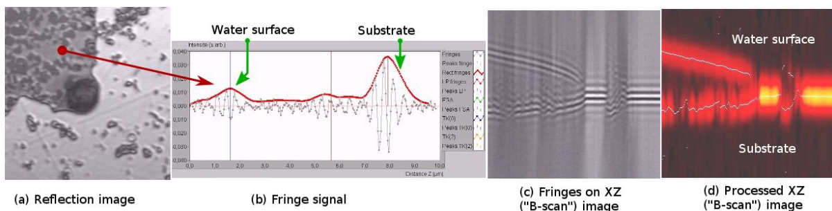
Figure 1. Exemple de mesure de la forme 3D d'une goutte d'eau sur une couche de colloïdes par la microscopie interférométrique (image 43x43 \mu\text{m} )
